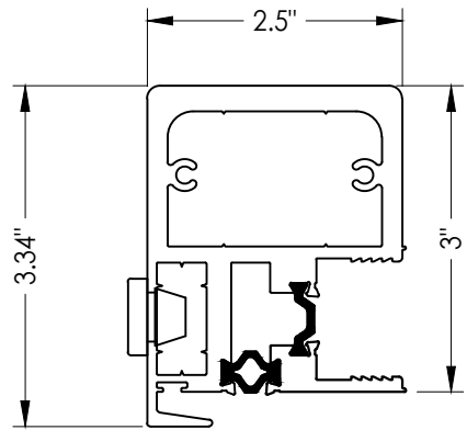
9 HP INTERLOCK
